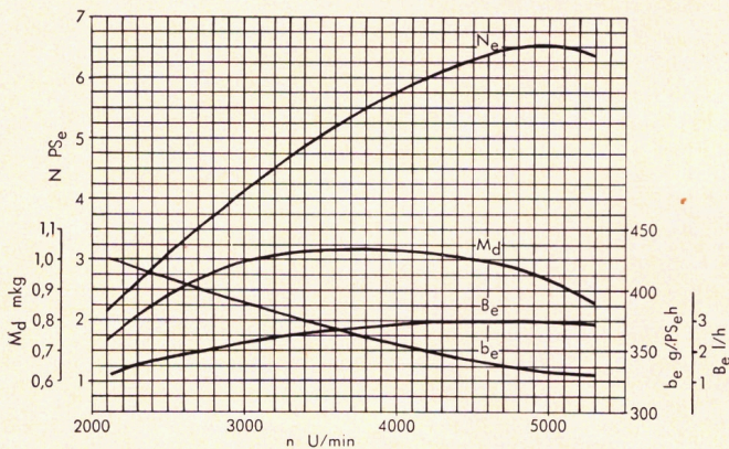
Motor-Kennlinien
